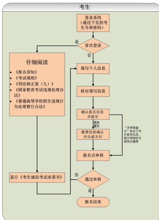
图 1.1 业务流程图
